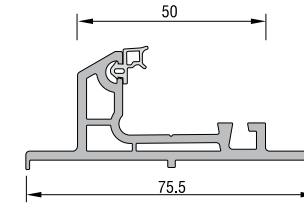
ÇİFT RAY ADAPTÖR PROFİLİ KODU: 22206 - 14000
