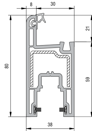
KANAT KIL FİTİLLİ PROFİL KODU : 21108 - 15200 (BEYAZ)
