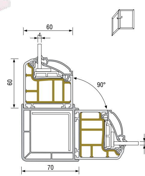
90° KÖŞE DÖNÜŞ PROFİLİ MONTAJ DETAYI
