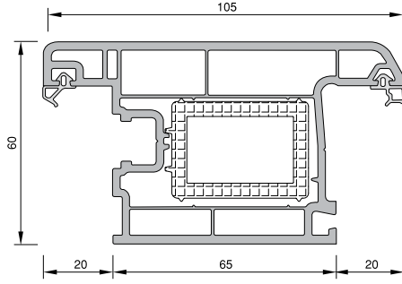
DİŞA AÇILIM KAPI KANAT PROFİLİ KODU : 21107 - 18100 (BEYAZ) CRP KODU : 71107 - 18100 (BEYAZ)
