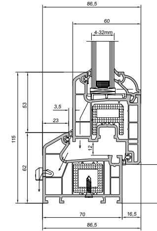
Kasa, Kanat Uygulaması
