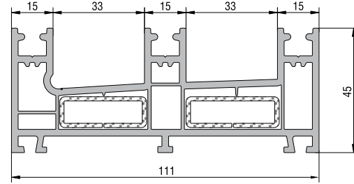
KASA PROFİLİ (ÜÇ RAY) KODU : 21108 - 01100 (BEYAZ)
