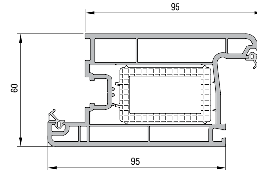
KAPI KANAT PROFİLİ KODU : 21107 - 17100 (BEYAZ) CRP : 71107 - 17100 (BEYAZ)
