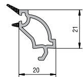
TEK CAM ÇİTASI (4 mm) KODU : 20101 - 04300 (BEYAZ)
