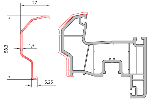
ALM. GİYDİRME FUGALI KANAT PRF. ELOKSAL (3902) KODU : 34025 - 28040
