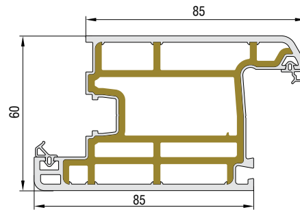
KAPI KANAT PROFİLİ KODU : 74107 - 17100 (BEYAZ)
