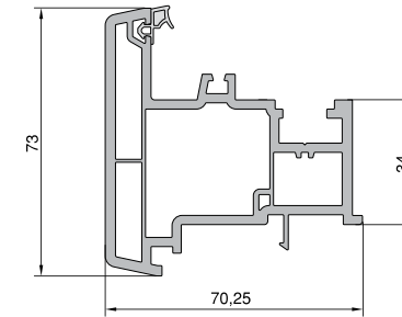
HAREKETLİ ORTA KAYIT PROFİLİ
