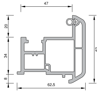
ÇİFT KANAT ARA PROFİLİ 22107-19000 (BEYAZ)
