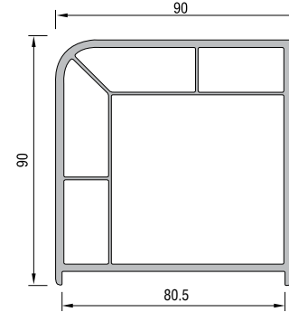
90° KÖŞE DÖNÜŞ PROFİLİ
