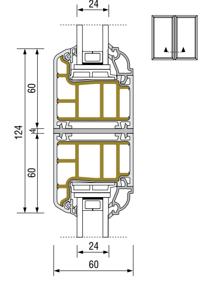
İNCE BİRLEŞTİRME PROFİLİ MONTAJ DETAYI
