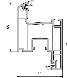
KANAT PROFİLİ KODU : 21105 - 15100 (BEYAZ)
