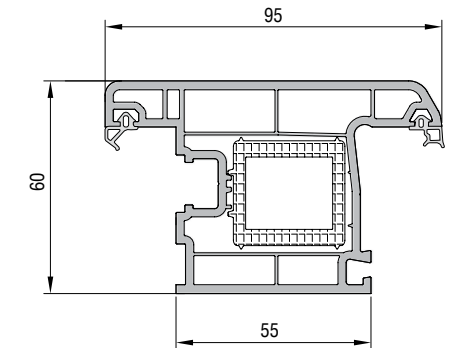
EKO DIŞA AÇILIM KAPI KANAT PROFİLİ KODU : 21107 - 18200 (BEYAZ) CRP : 71107 - 18200 (BEYAZ)
