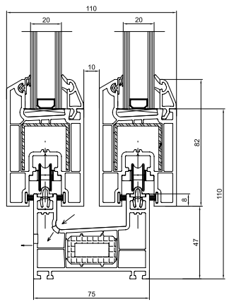
Eco Sürme Çift Ray Kasa - Kanat Montajı
