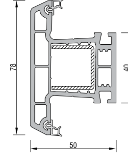
ORTA KAYIT PROFİLİ KODU: 21105 - 13000 (BEYAZ)
