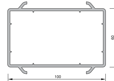
(60 X 100) TIRNAKLI KUTU KODU : 20104 - 06100 (BEYAZ)
