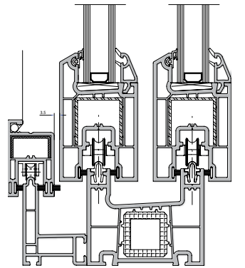
Sineklik Adaptörü Sürme Kasa Kanat Montajı
