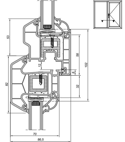
Orta Kayıt, Kanat Uygulaması
