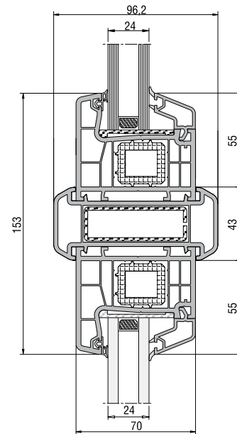
Geniş Bağ Profili Uygulaması
