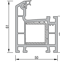
232 KASA PROFİLİ KODU: 21105 - 11000 (BEYAZ)
