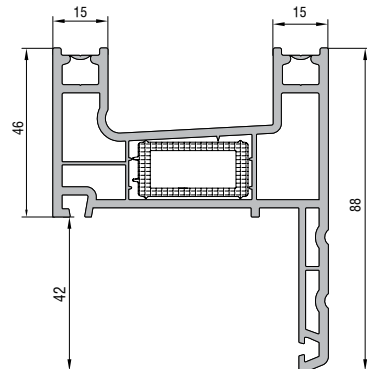
PERVAZLI KASA KODU : 21106 - 01100 (BEYAZ) CRP KODU: 71106 - 01100 (BEYAZ)
