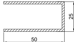
KAPI KANAT DESTEK SACI KODU : 34022 - 12012 KALINLIK : 1,2 mm
