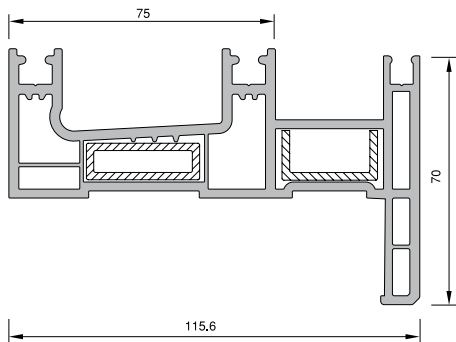
SİNEKLİKLİ SÜRME KASA KODU : 21409 - 01000 (BEYAZ) CRP KODU: 71409 - 01000 (BEYAZ)
