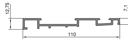
Alm. eşik ikinci Kanat Ray KODU: AD16 - 025
