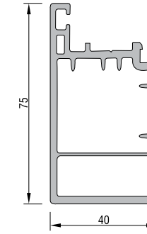
KANAT PROFİLİ 21601 - 01000 : BEYAZ
