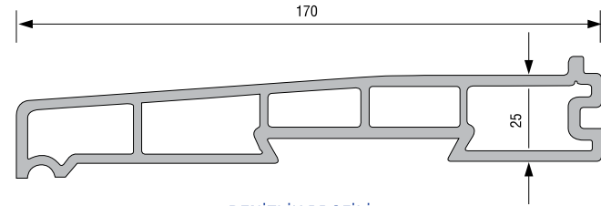
DENİZLİK PROFİLİ 20110 - 01000 : BEYAZ
