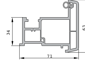
ÇİFT KANAT ARA PROFİLİ
