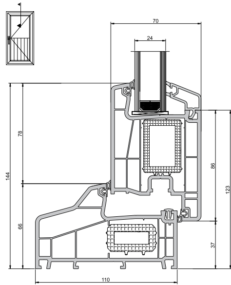
Kasa, Kapı Kanat Uygulaması
