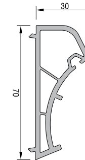
AÇILI DÖNÜŞ ADAPTÖRÜ KODU : 20111 - 04000
