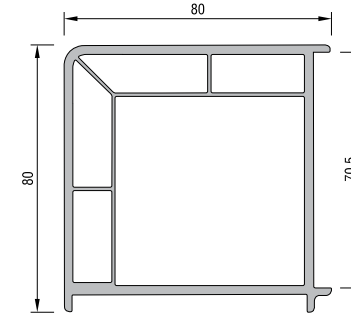
90° KÖŞE DÖNÜŞ PROFİLİ KODU : 20111 - 02000 (BEYAZ)
