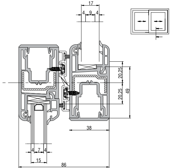
Sürme Kanat Ara Bindirme Uygulaması
