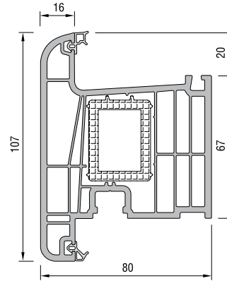
DIŞA AÇILIM KAPI KANAT PROFİLİ
