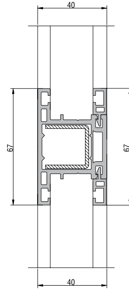
KEPEK ORTA KAYIT LAMEL UYGULAMASI
