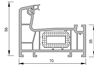
EKO KASA PROFİLİ
