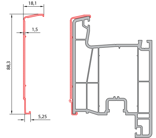
ALM. GİYDİRME KAPI KANAT PRF. ELOKSAL (3897) KODU : 34025 - 28060
