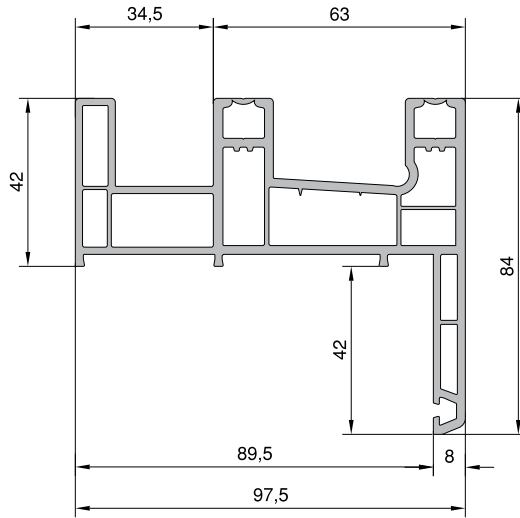
SÜRME PERVAZLI SİNEKLİK KASA KODU : 21108 - 01200 / 1.620
