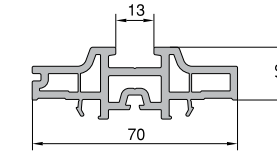
Hebeşibe Kanat ve Ray Adaptörü KODU: 20107 - 06000
