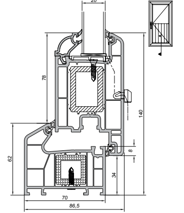
Kasa, D. Açılım Kapı Kanat Uygulaması
