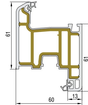
KANAT PROFİLİ KODU : 74107 - 15100 (BEYAZ)
