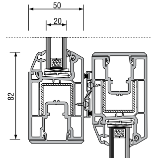
Sürme Arabindirme Montajı
