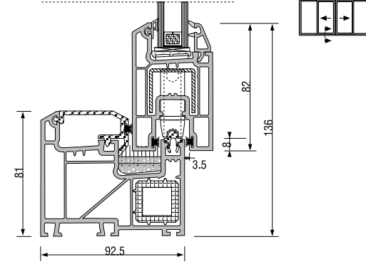
Sürme Tek Ray Kasa - Kanat Montajı
