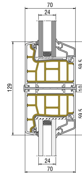
Bağlantı Profili Uygulaması
