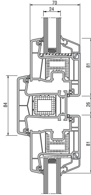
Kanat Ortakayıt Kanat Uygulaması
