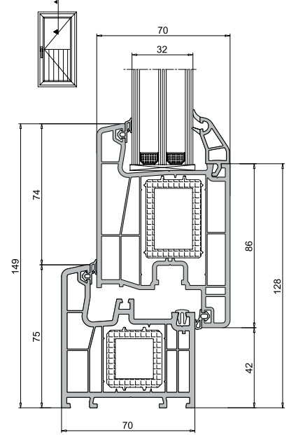
Kasa, Kapı Kanat Uygulaması
