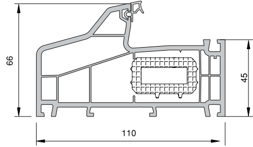
KASA PROFİLİ
