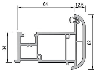
ÇİFT KANAT ARA PROFİLİ
