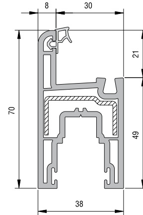
KODU : 21108 - 15000
