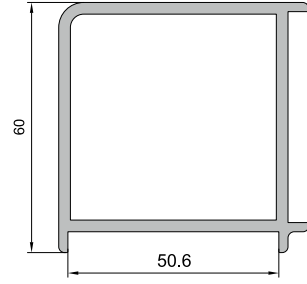
90° KÖŞE DÖNÜŞ PROFİLİ KODU : 20105 - 02000 (BEYAZ)
