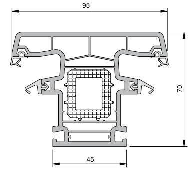
ORTA KAYIT PROFİLİ
