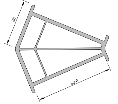
135° KÖŞE DÖNÜŞ PROFİLİ KODU : 20106 - 03000 (BEYAZ)
