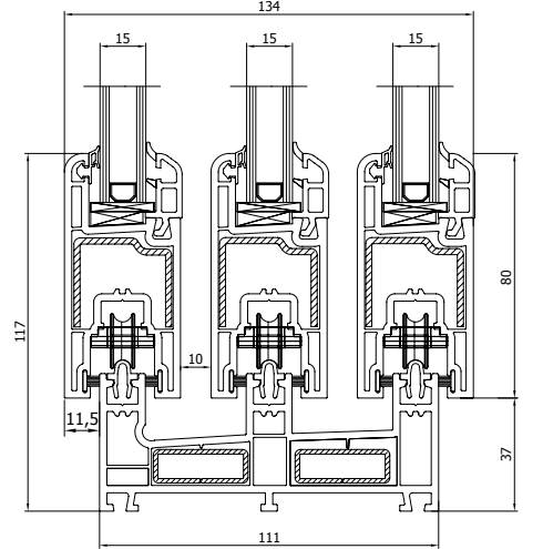
Üç Raylı Sürme Kasa Kanat Uygulaması
