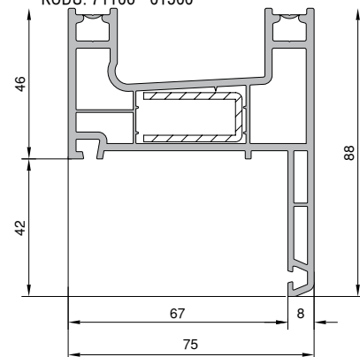
YENİ PERVAZLI KASA PROFİLİ KODU: 21106 - 01300 KODU: 71106 - 01300
