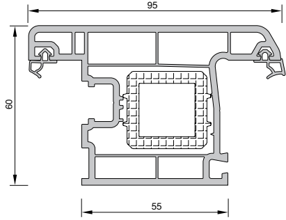
EKO DİŞA AÇILIM KAPI KANAT PROFİLİ KODU : 21107 - 18200 (BEYAZ) CRP KODU : 71107 - 18200 (BEYAZ)
