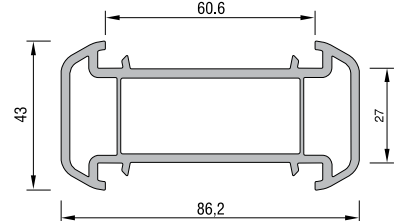
KALIN BAĞ PROFİLİ KODU : 20105 - 05200 (BEYAZ)
