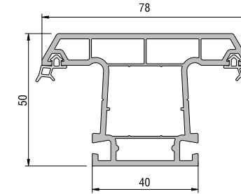
ORTA KAYIT PROFİLİ KODU : 21105 - 13100 (BEYAZ)
