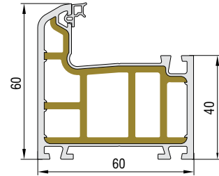
KASA PROFİLİ KODU : 74107 - 11100 (BEYAZ)
