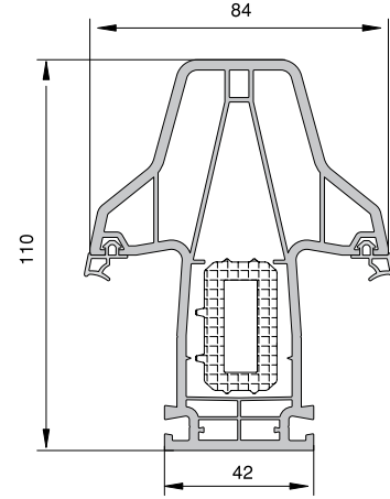
ORTA KAYIT PROFİLİ
