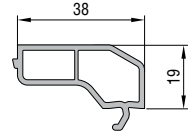
PVC KAPAMA PROFİLİ KODU: 20107 - 01200 BEYAZ
