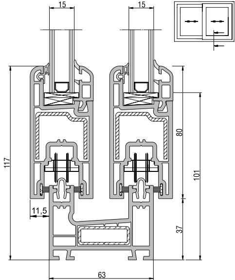
Sürme Kasa - Sürme Kanat Uygulaması
