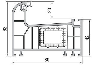
EKO KASA PROFİLİ
