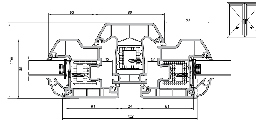
Kasa, Orta Kayıt, Kanat Uygulaması
