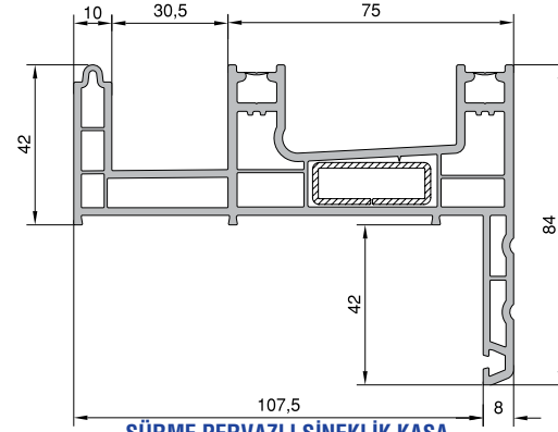
SÜRME PERVAZLI SİNEKLİK KASA KODU: 21106 - 01500 KODU: 71106 - 01500
