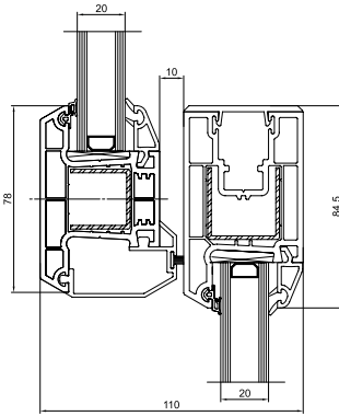
Sürme Ortakayıt - Kanat Montajı
