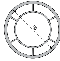
AÇILI DÖNÜŞ BORUSU (Ø 50) KODU : 20105 - 05100 (BEYAZ)
