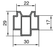
Sabit Kanat Yataklama Alm. (5cm) KODU: AD16 - 021
