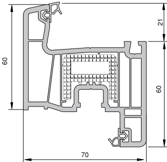
KANAT PROFİLİ
