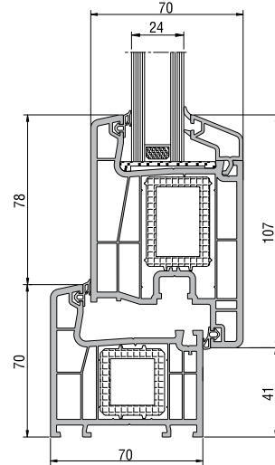
Kasa Kapı Kanat Uygulaması
