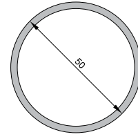
PVC BORU PROFİLİ (Ø 50) KODU : 20105 - 05000 (BEYAZ)
