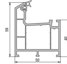
KASA PROFİLİ KODU : 21105 - 11100 (BEYAZ)
