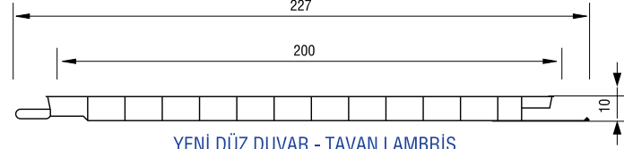
YENİ DÜZ DUVAR - TAVAN LAMBRİSİ 20103 - 01100 : BEYAZ
