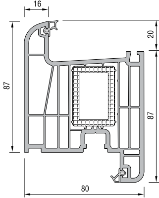
KAPI KANAT PROFİLİ
