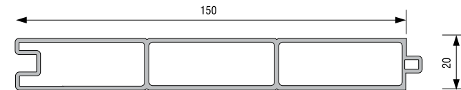
LAMBRI PROFİLİ 20102 - 01000 : BEYAZ
