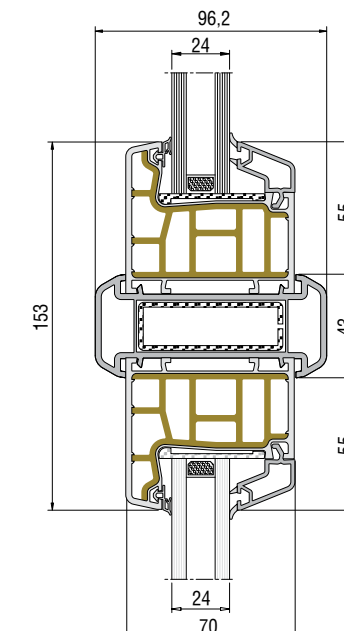
Geriş Bağlantı Profili Uygulaması
