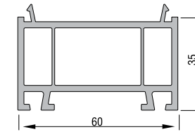
KASA YÜKSELTME PROFİLİ KODU : 20106 - 05000 (BEYAZ)
