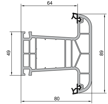
800 Seri O..Kayıt KODU: 21104 - 13300 KODU: 71104 - 13300
