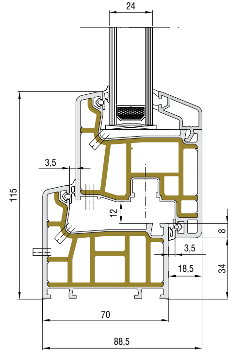
Kasa, Kanat Uygulaması
