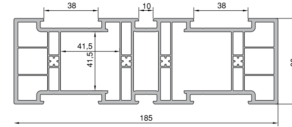
Hebeşibe Kasa KODU: 21104 - 11500
