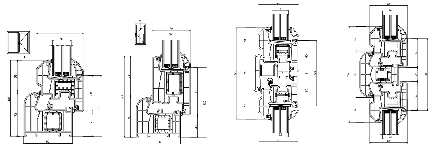
DAMLALIKLI KANAT & ORTA KAYIT MONTAJ DETAYI
