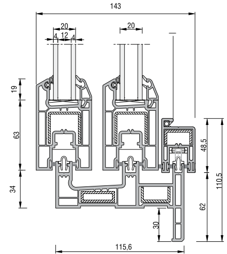
İç Sineklik Raylı Pervazlı Sürme Kasa Kanat Montajı
