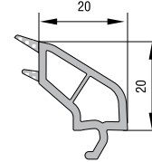
DÜZ CAM ÇİTASI (20 mm) KODU : 20101 - 04700 (BEYAZ)
