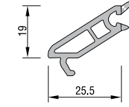
TEK CAM ÇİTASI (4 mm) 20101 - 03100 (BEYAZ)
