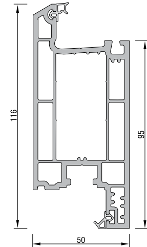
KAPI KANAT PROFİLİ KODU : 21105 - 17000 (BEYAZ)
