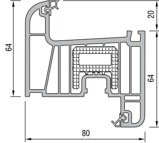
KANAT PROFİLİ
