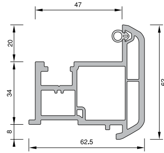
ÇİFT KANAT ARA PROFİLİ KODU : 22107 - 19000 (BEYAZ)
