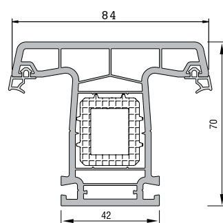
ORTA KAYIT PROFİLİ
