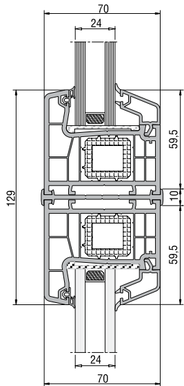
Bağ Profili Uygulaması
