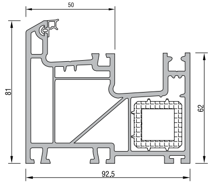
KASA PROFİLİ (Tek Ray) KODU : 21106 - 12000 (BEYAZ) CRP KODU: 71106 - 12000 (BEYAZ)
