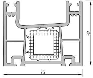
SÜPER KASA PROFİLİ (Çift Ray) KODU : 21106 - 01000 (BEYAZ) CRP KODU: 71106 - 01000 (BEYAZ)
