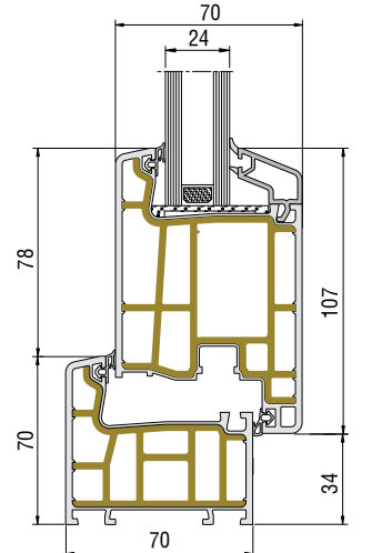
Kasa, Kapı Kanat Uygulaması
