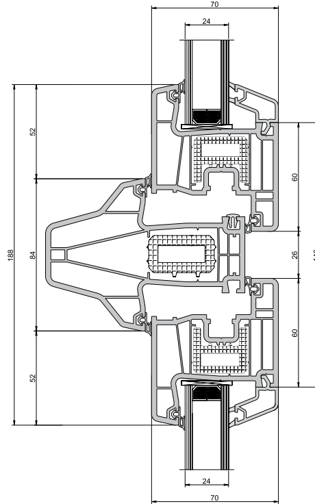
Kanat Orta Kayıt Uygulaması
