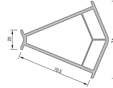
135° KÖŞE DÖNÜŞ PROFİLİ KODU : 20111 - 03000 (BEYAZ)
