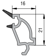
DEKORATİF ISI CAM ÇİTASI (24 mm) KODU : 20101 - 04500 (BEYAZ)
