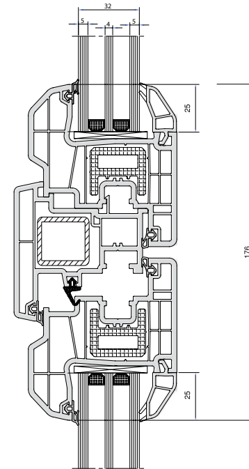
Hareketli Ortakayıt Damlalıklı Kanat uygulaması
