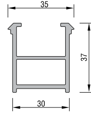
KASA MONTAJ PROFİLİ KODU : 20105 - 05300 (BEYAZ)
