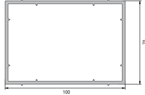
KASA 70X100 KUTU PROFİLİ KODU : 20111 - 06000 (BEYAZ)
