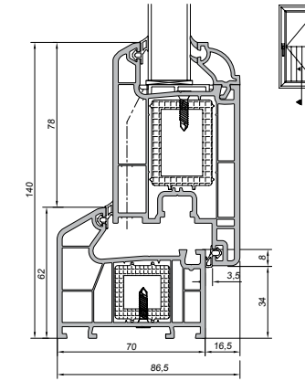
Kasa, Kapı Kanat Uygulaması
