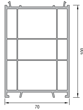
KASA YÜKSELTME PROFİLİ KODU : 20111 - 08100 (BEYAZ)
