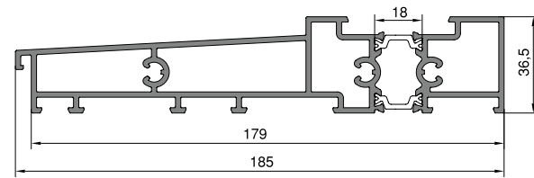
Hebeşibe Isı Yalıtımlı Alm. eşik Profili KODU: AD16 - 027
