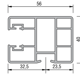
PANJUR YENİ YAN RAY 21501 - 04100 (BEYAZ)
