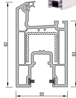
SÜRME KANAT PROFİLİ KIL FITİLLİ KODU: 22106 - 15300 / 6.50
