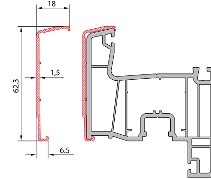
ALM. GİYDİRME NORMAL KANAT PRF. ELOKSAL (3898) KODU : 34025 - 28030
