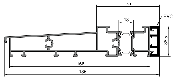
Hebeşibe İç Kısmı PVC Isı Yalıtımlı Alm. eşik Prf. KODU: AD16 - 026
