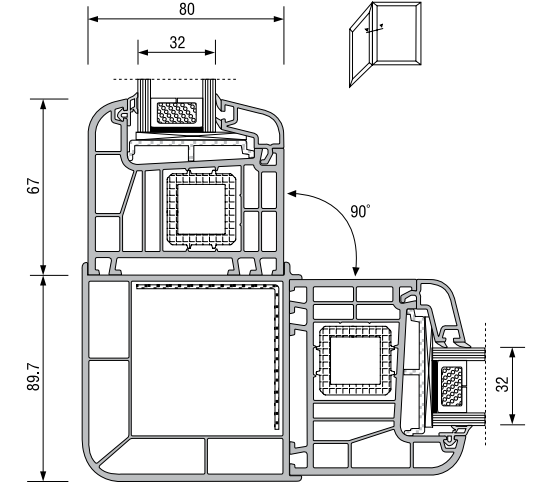
90° Köşe Profili Montajı
