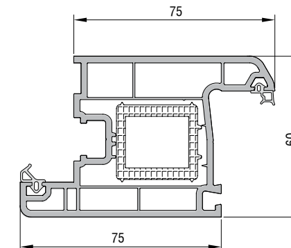
KAPI KANAT PROFİLİ KODU : 21107 - 17100 (BEYAZ) CRP : 71107 - 17100 (BEYAZ)
