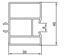
ALM. RAY ALTI SİNEKLİK ADAPTÖRÜ KODU : 21108 - 01000 (BEYAZ)
