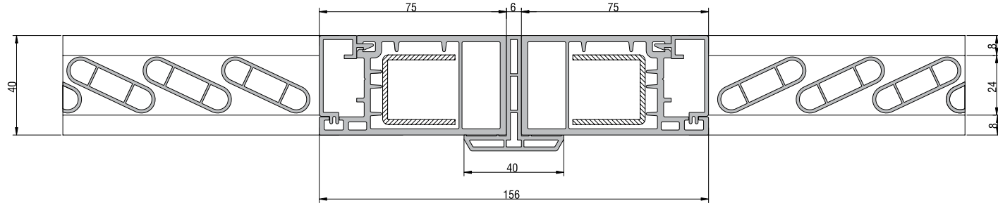
KEPEK KANAT T PROFİLİ UYGULAMASI
