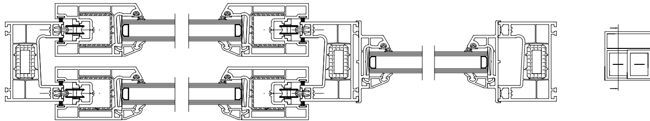
Çift ray Sürme Sistemi Üst Sabit Alt Hareketli Sürme Montajı
