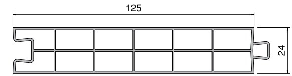
125x24 LAMBRI PROFİLİ 20102 - 05000 : BEYAZ
