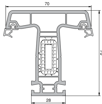
DAR ORTA KAYIT PROFİLİ
