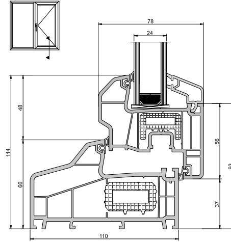
Kasa Damlalıklı Kanat Uygulaması
