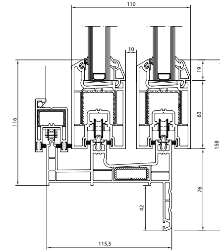
Dış Sineklik Raylı İç Pervazlı Sürme Kasa Kanat Montajı
