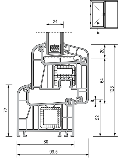
Kasa Kanat Montajı
