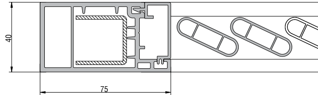
KEPEK KANAT LAMEL UYGULAMASI
