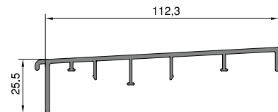
Alm.Eşik Kapama KODU: AD16 - 024
