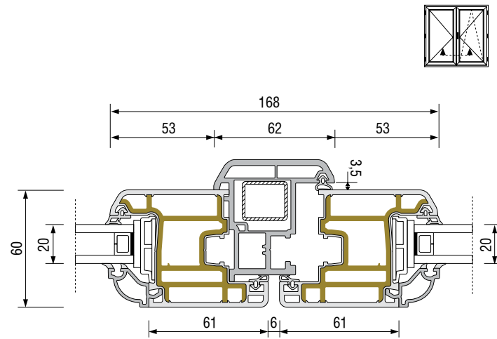
HAREKETLİ ORTA KAYIT & KANAT MONTAJ DETAYI
