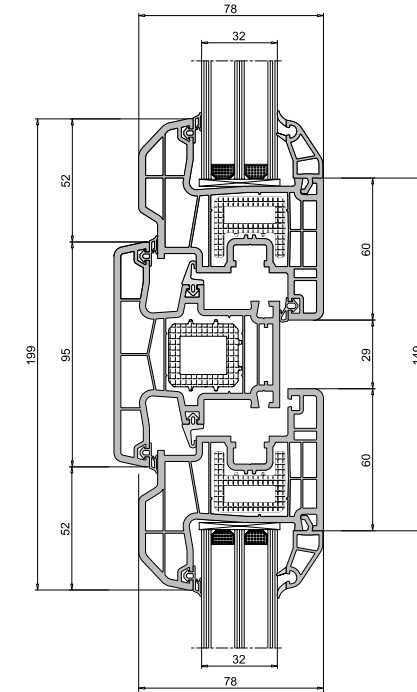
Damlalıklı Kanat Ortakayıt Ortakayıt Damlalıklı Kanat Uygulaması
