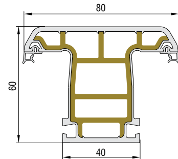
ORTA KAYIT PROFİLİ KODU : 74107 - 13100 (BEYAZ)
