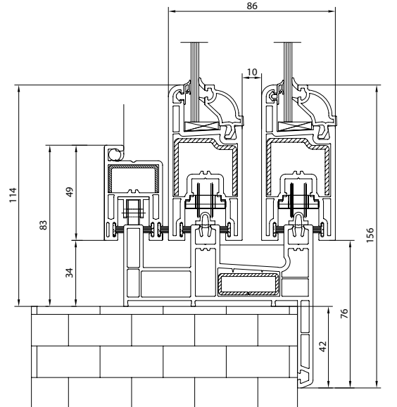
Sineklikli Pervazlı Kasa Kanat Uygulaması
