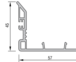
YENİ SÜRME ALIN KAPAMA PROFİLİ KODU: 22107 - 01100 / 6.50
