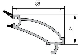
DEKORATİF TEK CAM ÇİTASI (4 mm) KODU : 20101 - 04400 (BEYAZ)
