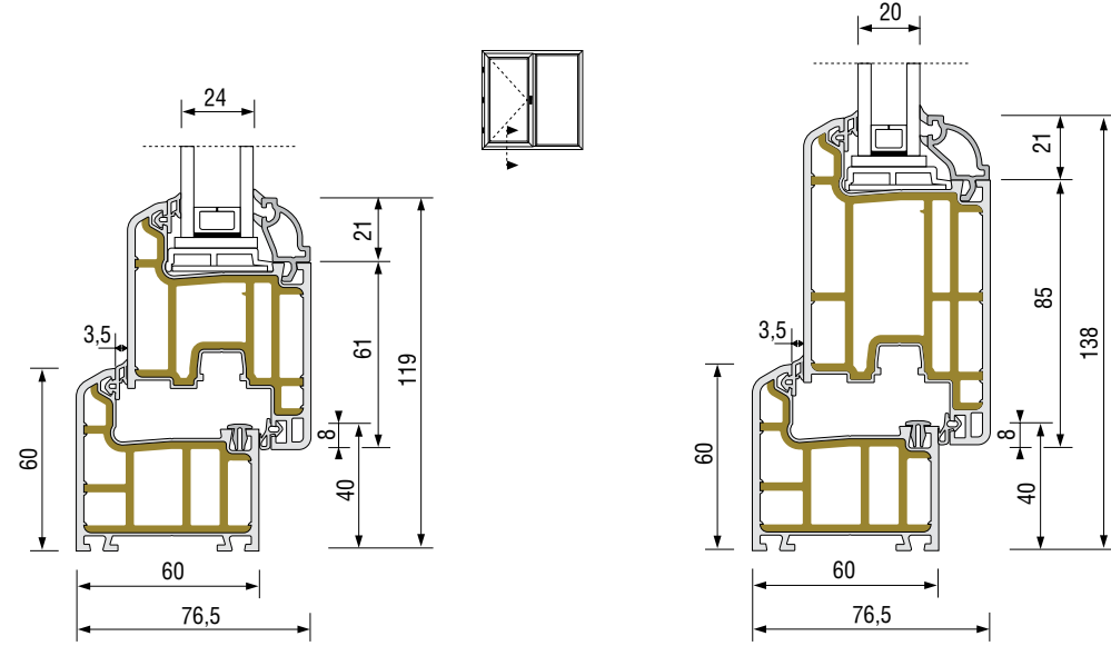
KASA KANAT MONTAJ DETAYI
