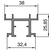
Kanat Üst Ray Alm. KODU: AD16 - 019
