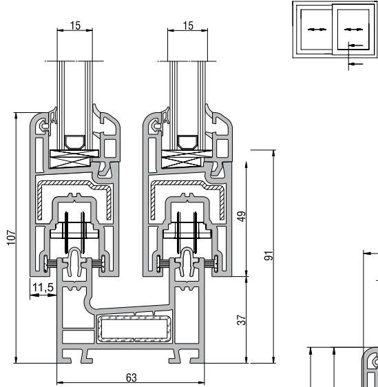
Sürme Kasa - Eco Sürme Kanat Uygulaması
