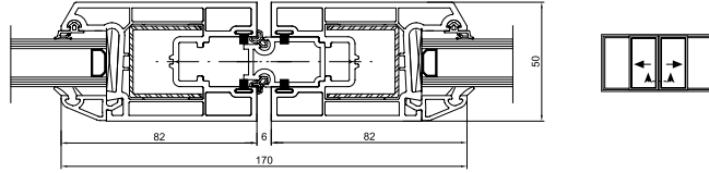
Sürme Çift Kanat Birleşim Montajı
