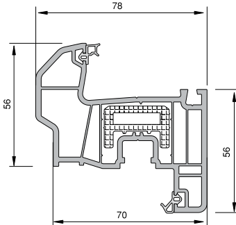
DAMLALIKLI KANAT PROFİLİ
