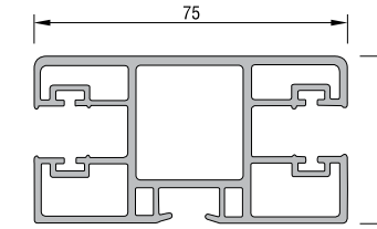
PANJUR ORTA YAN RAY 21501 - 05000 (BEYAZ)
