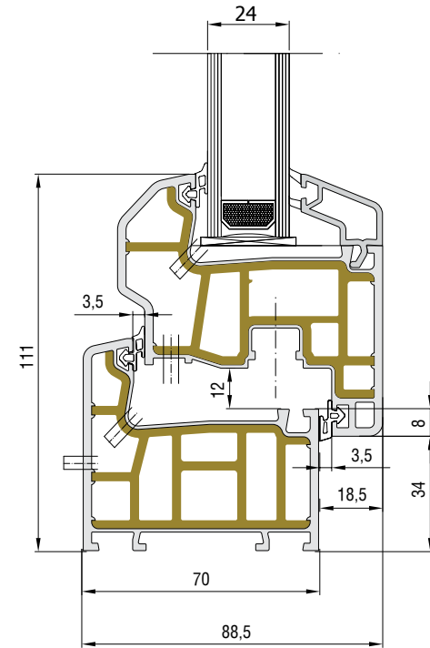
Kasa, Damlalıklı Kanat Uygulaması
