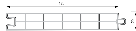
125'lik İKİ ODACIKLI LAMBRI PROFİLİ 20102 - 04000 : BEYAZ
