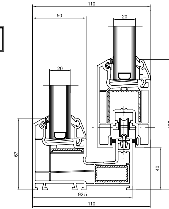
Yeni Sürme Tek Ray Kasa - Kanat Montajı
