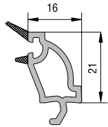
DEKORATİF ISI CAM ÇİTASI (24 mm) KODU : 20101 - 04500 (BEYAZ)
