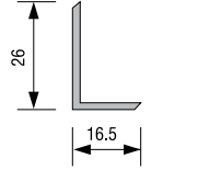
PVC L PROFİLİ (GENİŞ) 20110 - 06000 : BEYAZ
