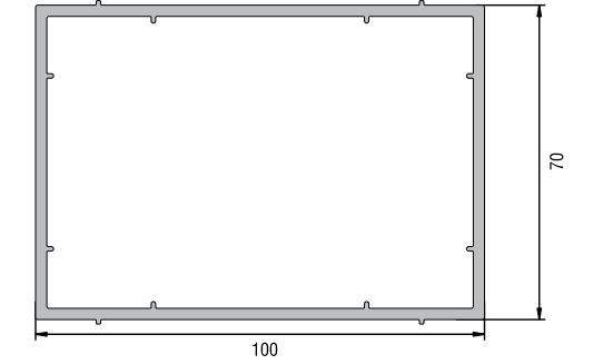
KASA 70X100 KUTU PROFİLİ KODU : 20111 - 06000 (BEYAZ)
