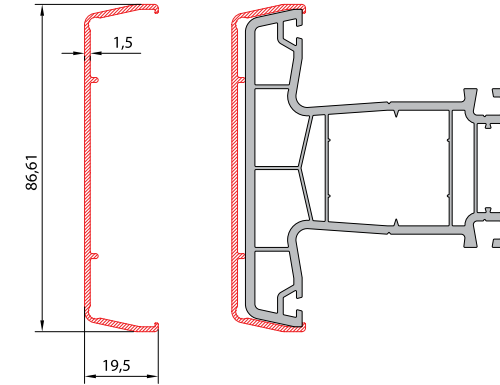
ALM. GİYDİRME ORTA KAYIT PRF. ELOKSAL (3899) KODU : 34025 - 28050
