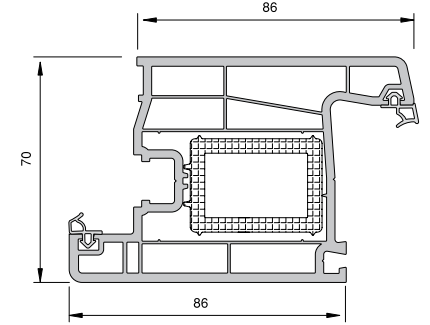
KAPI KANAT PROFİLİ
