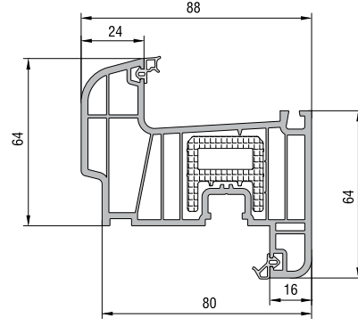
DAMLALIKLI KANAT PROFİLİ
