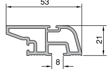
Hebeşibe Kanat Ara Bindirme KODU: 20107 - 07000
