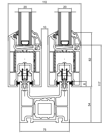
Sürme Çift Ray Kasa - Kanat Montajı
