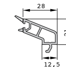
ÇİFT CAM ÇİTASI 20 mm
