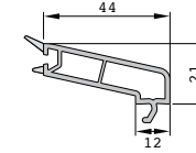
TEK CAM ÇİTASI 4-6 mm
