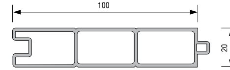
LAMBRI PROFİLİ 20102 - 02000 : BEYAZ
