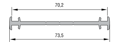
BAĞ PROFİLİ KODU : 20111 - 01100 (BEYAZ)
