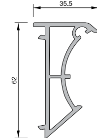
AÇILI DÖNÜŞ ADAPTÖRÜ KODU : 21106 - 04100 (BEYAZ)
