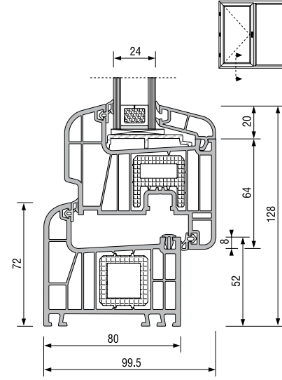
Kasa Damlalıklı Kanat Montajı
