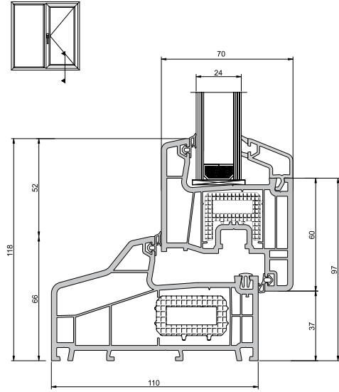
Kasa Kanat Uygulaması
