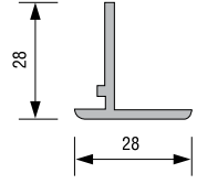
PVC T ÇİTASI 20110 - 05000 : BEYAZ
