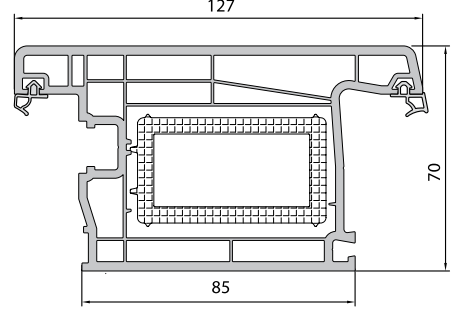
SÜPER DİŞA AÇILIM KAPI KANAT PROFİLİ
