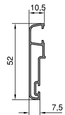
Kasa Dış Pervaz Alm. KODU: AD16 - 022
