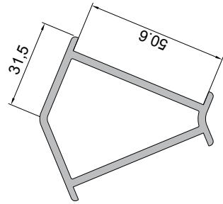
135° KÖŞE DÖNÜŞ PROFİLİ KODU : 20105 - 03000 (BEYAZ)
