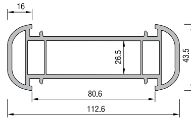
KALIN BAĞ PROFİLİ
