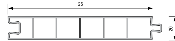
125'lik TEK ODACIKLI LAMBRI PROFİL 20102 - 03000 : BEYAZ
