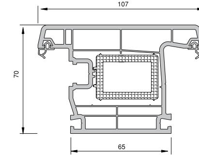
DİŞA AÇILIM KAPI KANAT PROFİLİ
