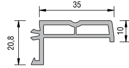
KASA KLİPS PERVAZ KODU : 20108 - 07000 (BEYAZ)
