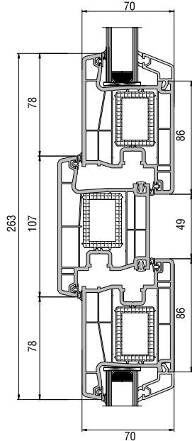
Kapı Kanat - Dışa Açılım Kapı Kanat Uygulaması
