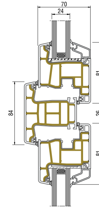
Kanat, Ortakayıt, Kanat Uygulaması
