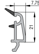
ÜÇ CAM ÇİTASI (32 mm) KODU : 20101 - 04600 (BEYAZ)
