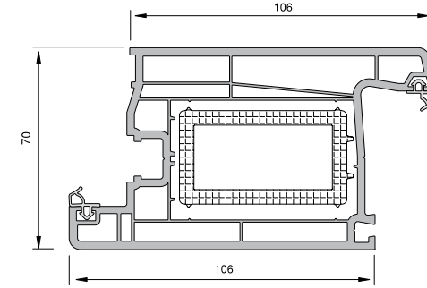
GENİŞ KAPI KANAT PROFİLİ
