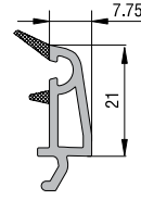
ÜÇ CAM ÇİTASI (32 mm) KODU : 20101 - 04600 (BEYAZ)
