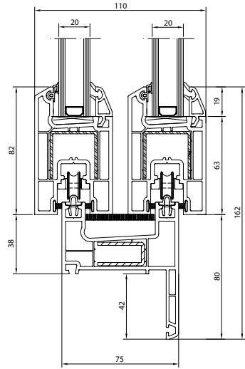
Düz Pervazlı Çift Ray Kasa - Kanat Montajı
