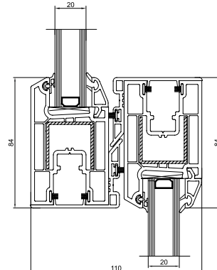
Yeni Sürme Kanat Arka Kapama Montajı
