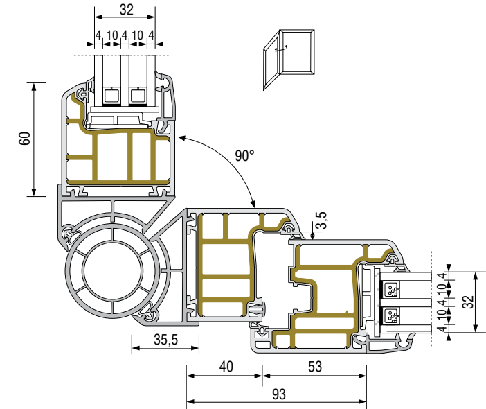
BORU PROFİLİ MONTAJ DETAYI
