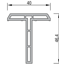
KEPENK T PROFİLİ 21601 - 06000 : BEYAZ
