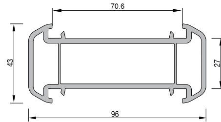
KALIN BAĞ PROFİLİ KODU : 20111 - 05000 (BEYAZ)
