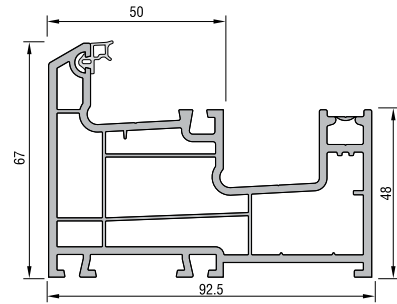
YENİ KASA PROFİLİ (Tek Ray) KODU: 21106 - 12100 (BEYAZ)
