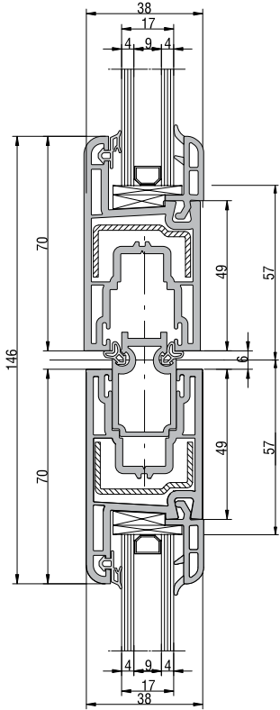
Sürme Kanat Uygulaması
