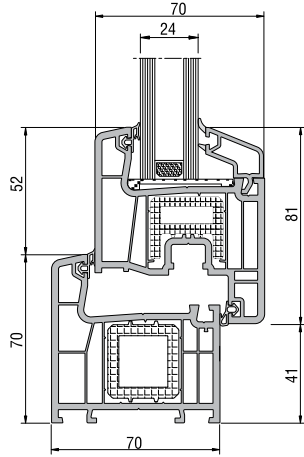
Kasa Kanat Uygulaması
