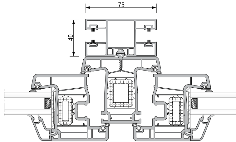
Orta Ray Uygulaması
