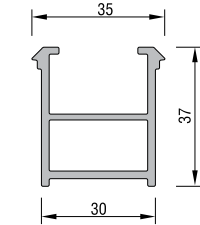
KASA MONTAJ PROFİLİ KODU : 20105 - 05300 (BEYAZ)
