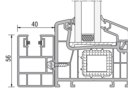
Yeni Yan Ray Uygulaması
