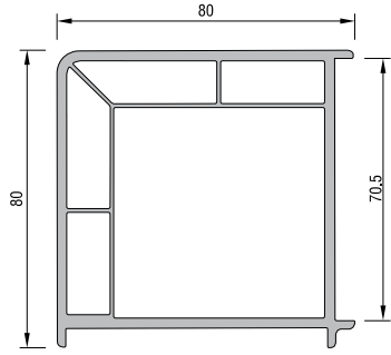
90° KÖŞE DÖNÜŞ PROFİLİ KODU : 20111 - 02000 (BEYAZ)
