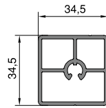
Kasa iç Çektirme Alm. (8cm) KODU: AD16 - 023
