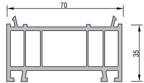
KASA YÜKSELTME PROFİLİ KODU : 20111 - 08000 (BEYAZ)
