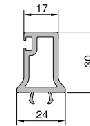
Hebeşibe Kasa Orta Adaptörü KODU: 20107 - 07100
