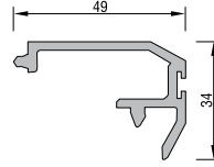
ALÜMİNYUM KAPAMA PROFİLİ KODU: 34025 - 13010 ELOKSAL
