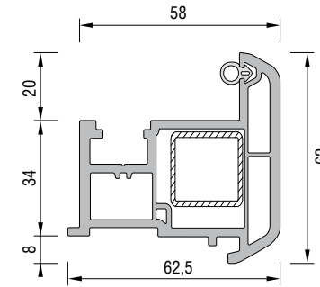
ÇİFT KANAT ARA PROFİLİ KODU : 22107 - 19000 (BEYAZ)
