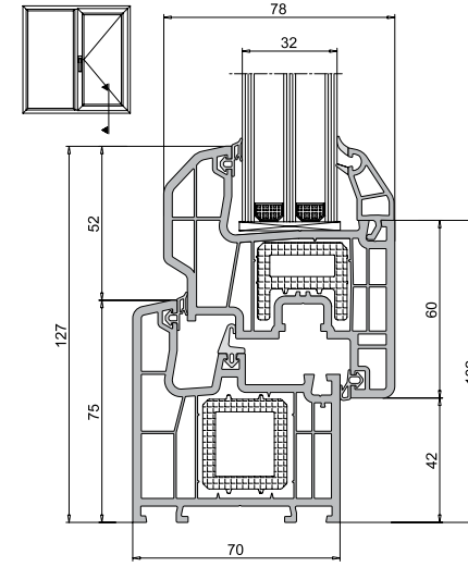
Kasa Damlalıklı Kanat Uygulaması
