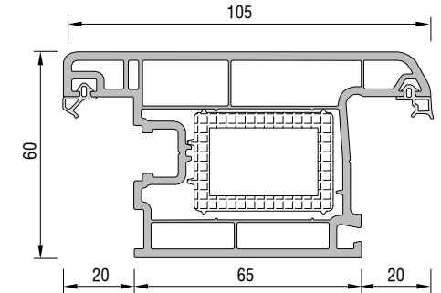
DIŞA AÇILIM KAPI KANAT PROFİLİ KODU : 21107 - 18100 (BEYAZ) CRP : 71107 - 18100 (BEYAZ)
