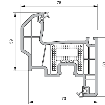
DAMLALIKLI KANAT PROFİLİ
