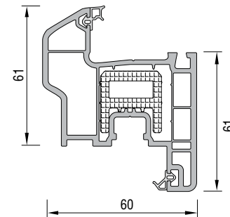
DAMLALIKLI KANAT PROFİLİ KODU : 21107 - 16100 (BEYAZ) CRP : 71107 - 16100 (BEYAZ)
