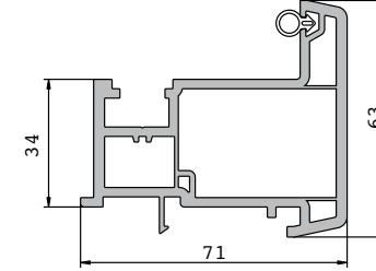
YENİ ÇİFT KANAT ARA PROFİLİ
