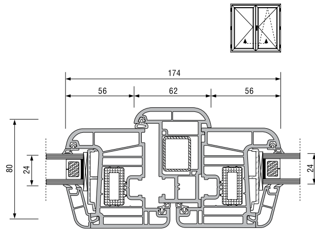
Hareketli Orta Kayıt Montajı
