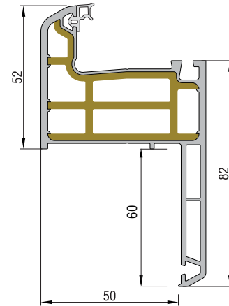
PERVAZLI KASA PROFİLİ KODU : 74107 - 11300 (BEYAZ)
