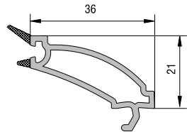
DEKORATİF TEK CAM ÇİTASI (4 mm) KODU : 20101 - 04400 (BEYAZ)
