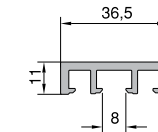
Alm.Eşik Arka Kapama KODU: 20107 - 02200
