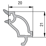
DEKORATİF ISI CAM ÇİTASI (20 mm) KODU : 20101 - 04300 (BEYAZ)
