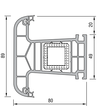
ORTA KAYIT PROFİLİ
