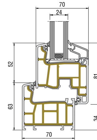
Kasa, Kanat Uygulaması
