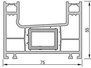
KASA PROFİLİ (Çift Ray) KODU : 21106 - 01400 (BEYAZ) CRP KODU: 71106 - 01400 (BEYAZ)
