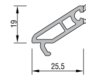
TEK CAM ÇİTASI KODU : 20101 - 03100 (BEYAZ)
