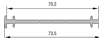
BAĞ PROFİLİ KODU : 20111 - 01100 (BEYAZ)
