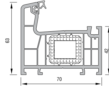
KASA PROFİLİ
