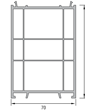
KASA YÜKSELTME PROFİLİ KODU : 20111 - 08100 (BEYAZ)
