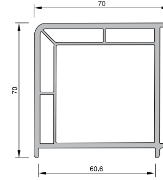
90° KÖŞE DÖNÜŞ PROFİLİ KODU : 20106 - 02000 (BEYAZ)
