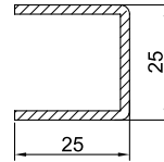
KASA, KANAT, ORTA KAYIT DESTEK SACI KODU : 34022 - 12003 KALINLIK : 1,2 mm
