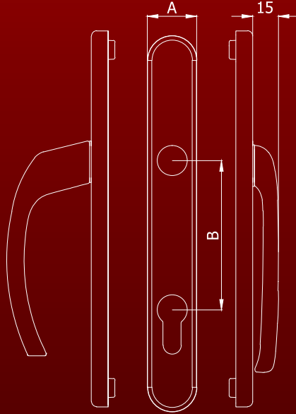
KATLANIR KAPI KOLU
