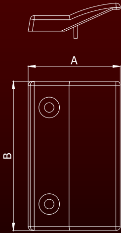
PVC DIŞ ÇEKME KOL
